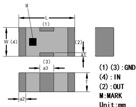
建议焊盘尺寸
